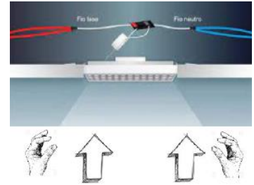
FIGURA (4) SUSPENDER A LUMINARIA PARA ENCAIXE NO NICHÔ.
