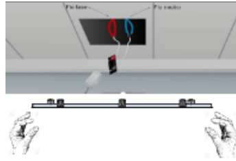
FIGURA (3) LIGAR O DRIVER AOS FIOS DE ENERGIA QUE SAEM DA SUPERFÍCIE. *FIO FASE *FIO NEUTRO AJUSTAR A MOLLA PARA ENCAIXE NO NICHÔ JÁ CORTADO.
