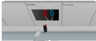
FIGURA (3) LIGAR O DRIVER AOS FIOS DE ENERGIA QUE SAEM DA SUPERFÍCIE. *FIO FASE *FIO NEUTRO AJUSTAR A MOLA PARA ENCAIXE NO NICHU JÁ CORTADO.
